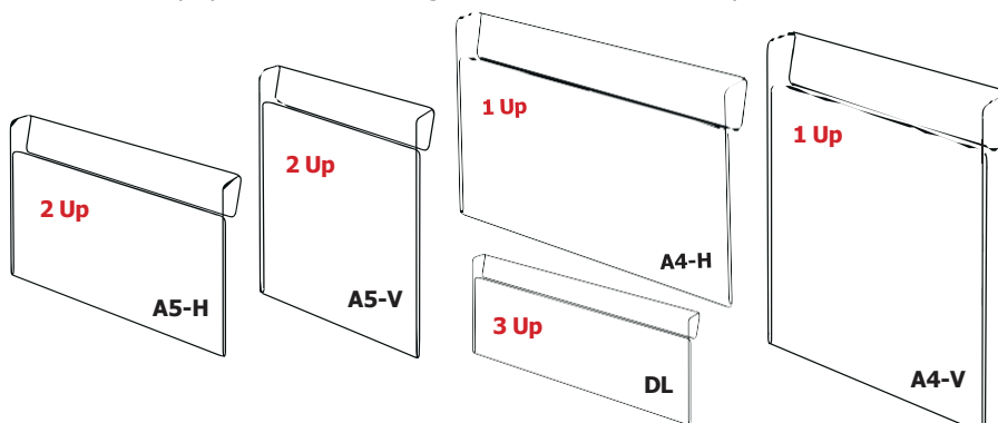
A5 - Horizontal - 215 x 157 x 20mm - ABHA5-H A5 - Vertical - 157 x 215 x 20mm - ABHA5-V DL - Horizontal - 215 x 105 x 20mm - ABHDL A4 - Horizontal - 300 x 215 x 20mm - ABHA4-H A4 - Vertical - 215 x 300 x 20mm - ABHA4-V
